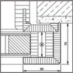
vor der Wand: Einlaufrichter
