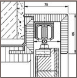
vor der Wand: Laufschiene
