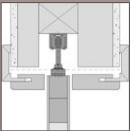
in der Wand: versetzter Sturz
